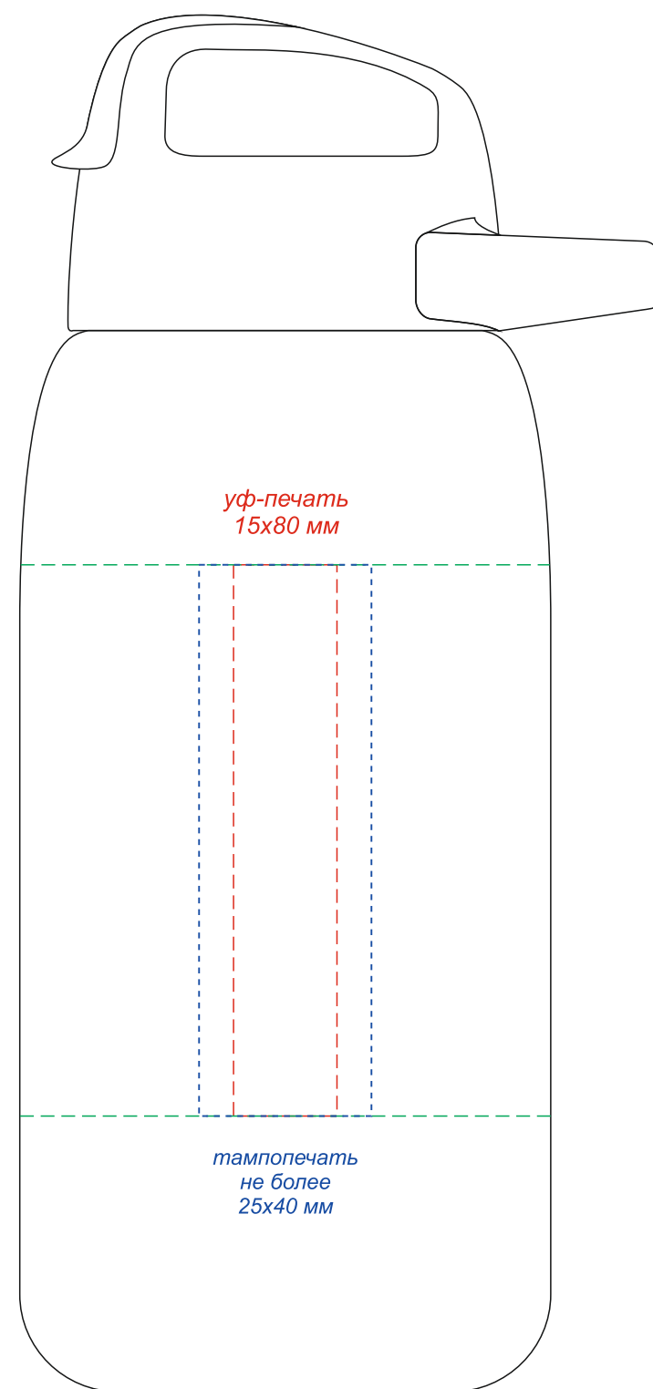
вид справа
