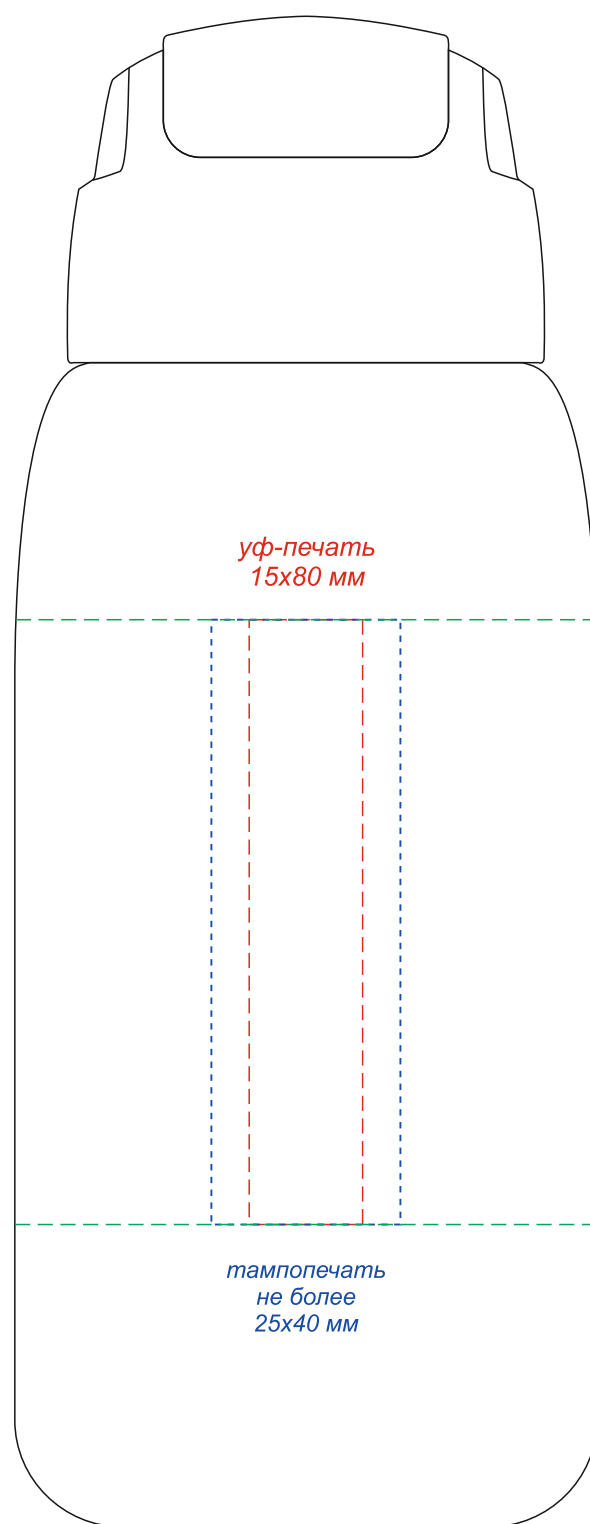
вид спереди
